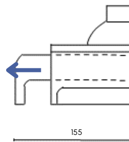
Asiento deslizable
