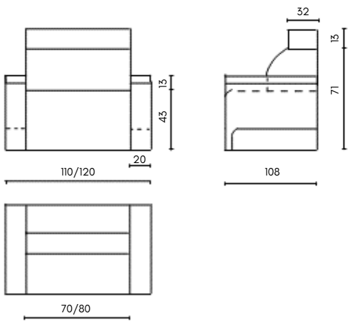
Brazo deslizable
